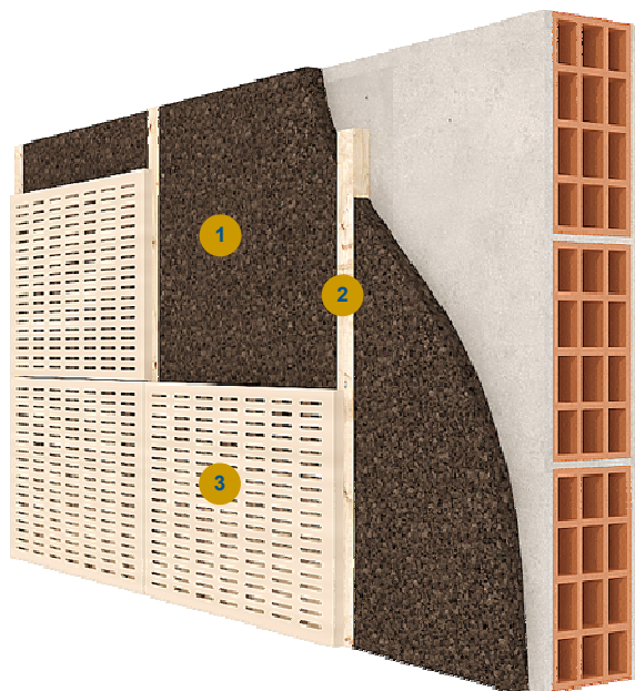
1 Aglomerado Negro de Corcho Expandido - ICB 2 Tableado 3 Paineles perforados
